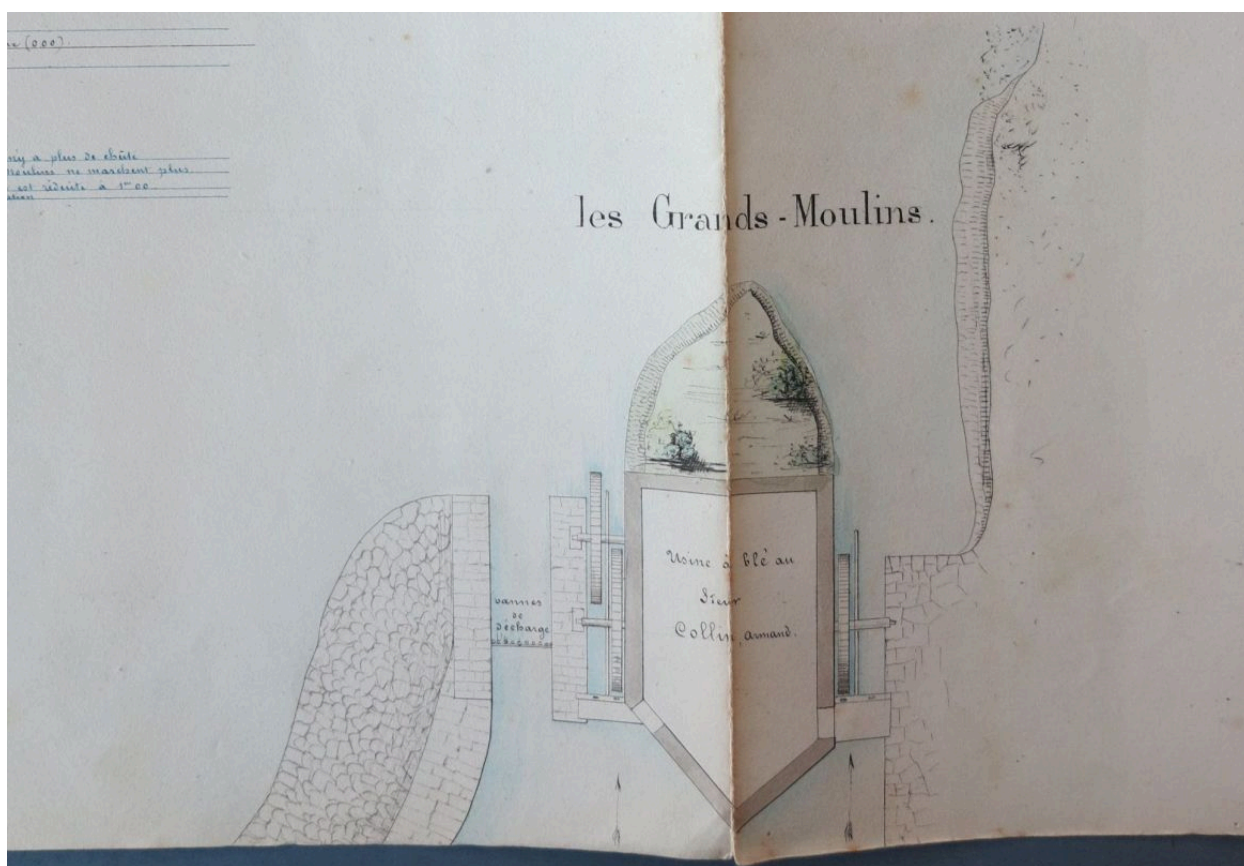
Les Grands-Moulins, usine à blé, plan par Delafons ingénieur, avril 1858.
