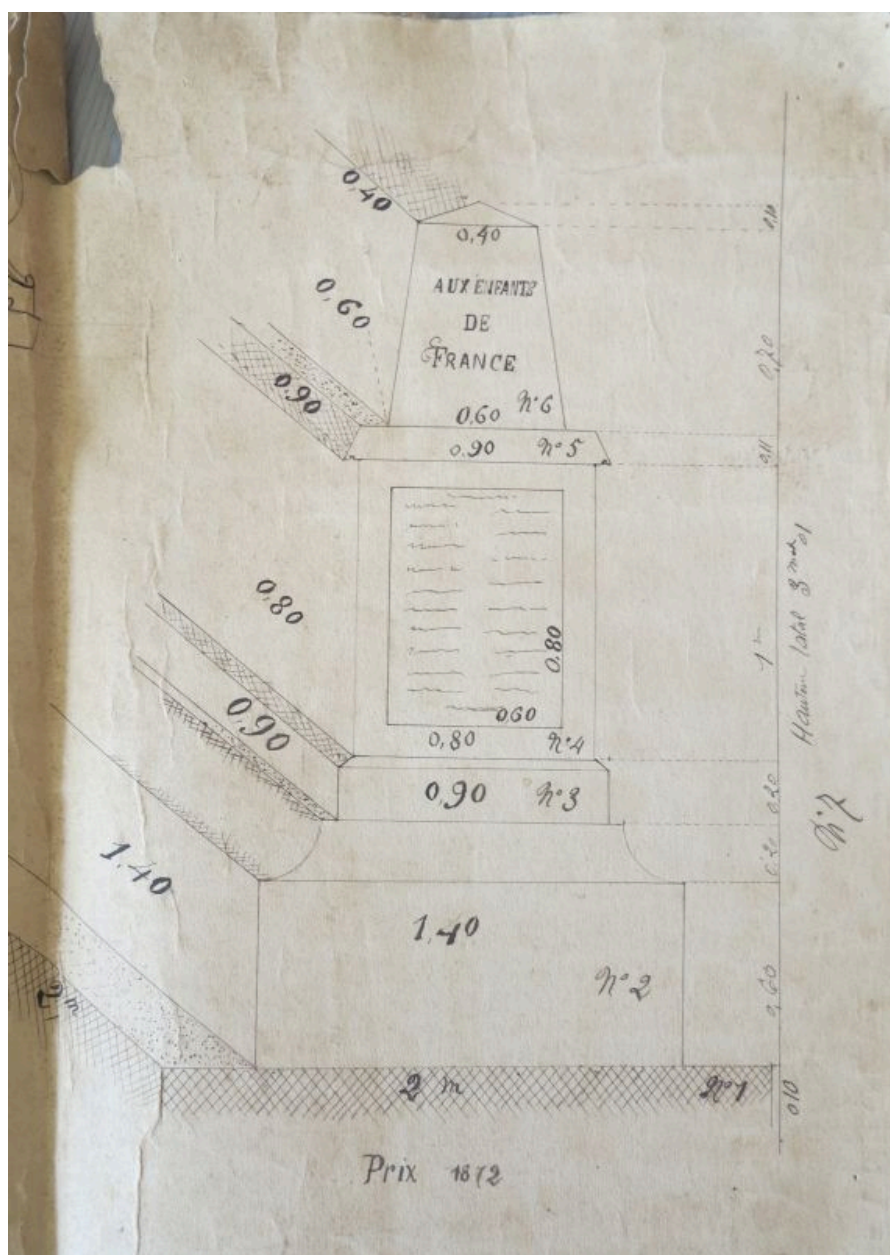
Plan coté du monument aux morts (archives municipales).
