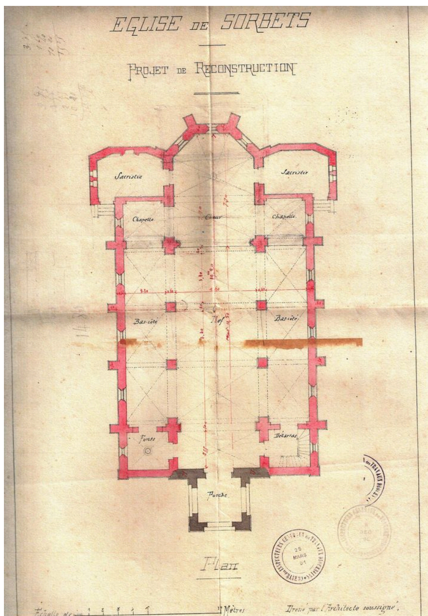
"Église de Sorbets, projet de reconstruction", par l'architecte Henri Depruneaux, 1891 (AM Sorbets) : plan.
