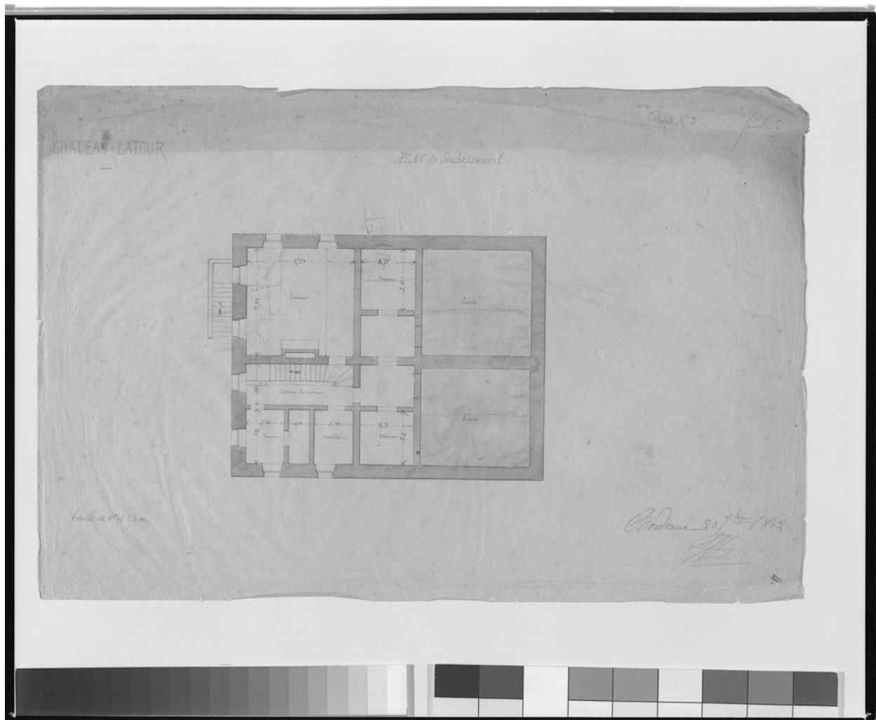
Projet de château, projet n°3 : plan du soubassement, feuille 2, par Henri Duphot, 20 septembre 1862 (conservé au château?).
