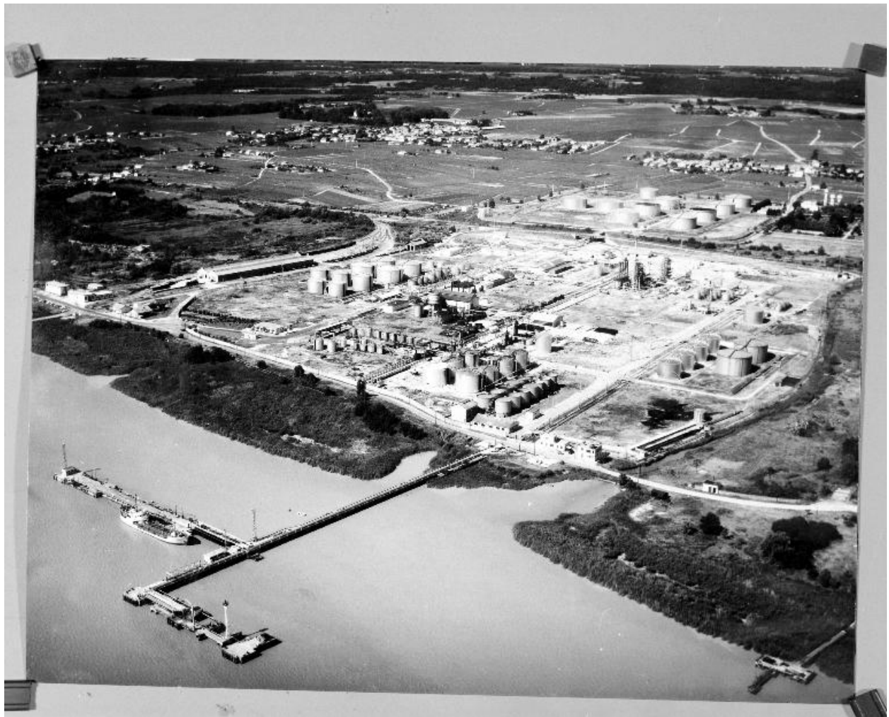
Photographie aérienne, en 1966 (collection particulière) : appontements pétroliers et vue d'ensemble de la raffinerie, depuis le nord-est.
