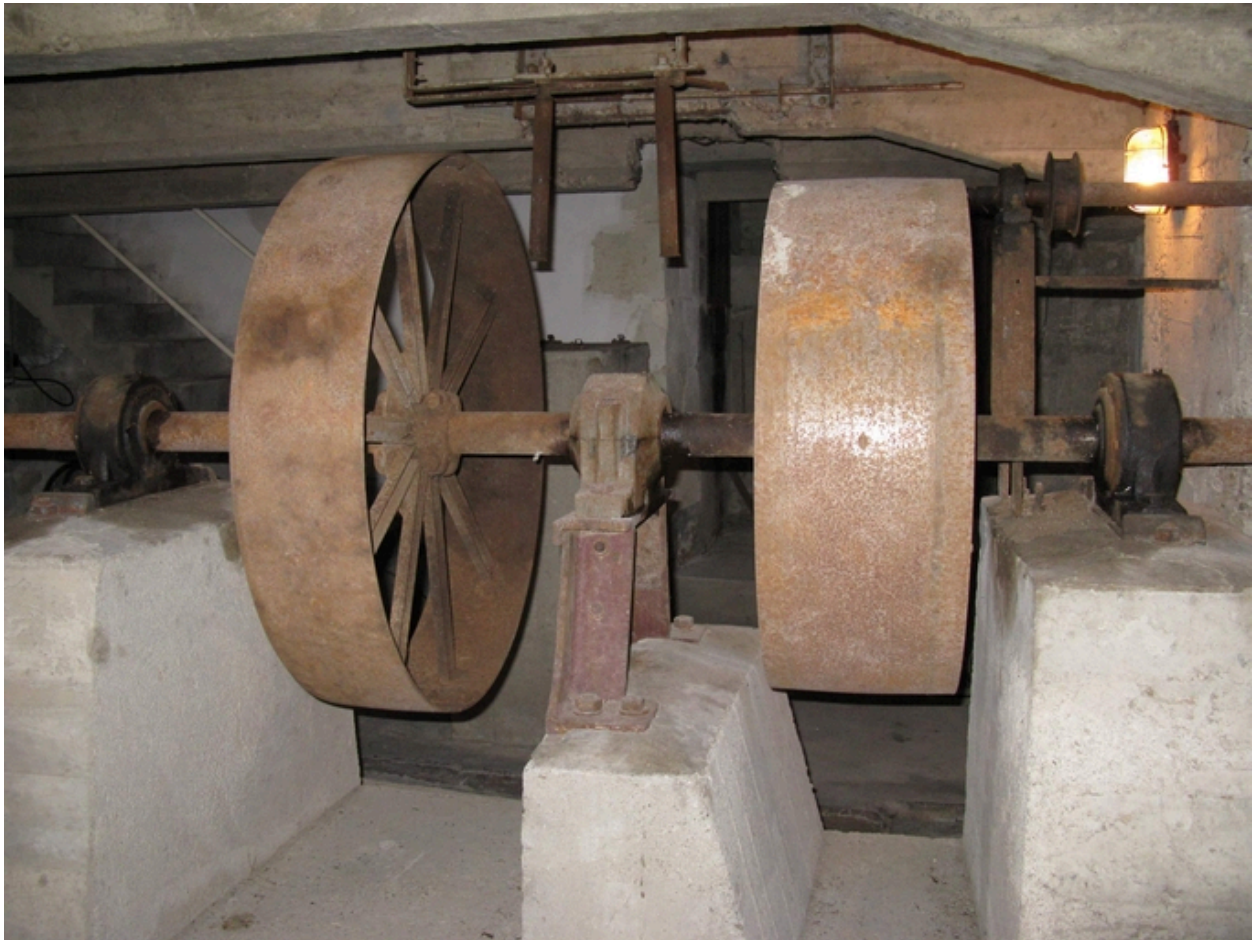
Etage de soubassement, organes de transmission.
