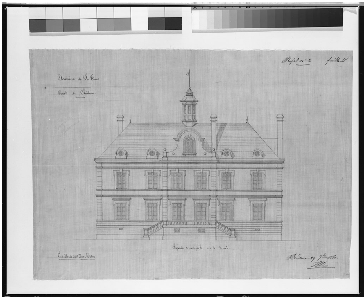
Projet de château, projet n°2 : façade principale sur la rivière, feuille 5, par Henri Duphot, 29 novembre 1860 (conservé au château?).
