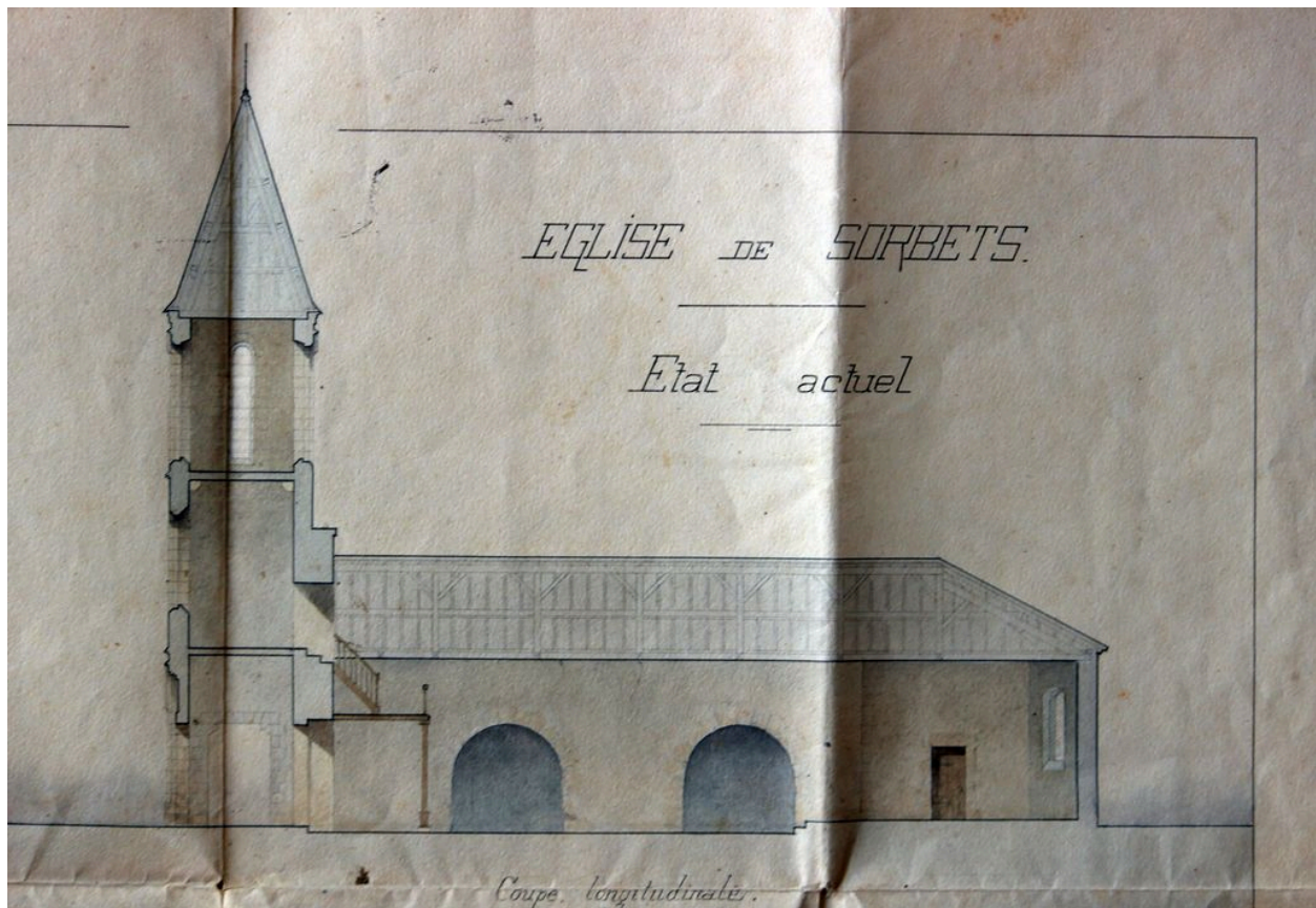
"Église de Sorbets, état actuel", relevés par l'architecte Henri Depruneaux, s.d. [1891] (AM Sorbets). Détail : coupe longitudinale.
