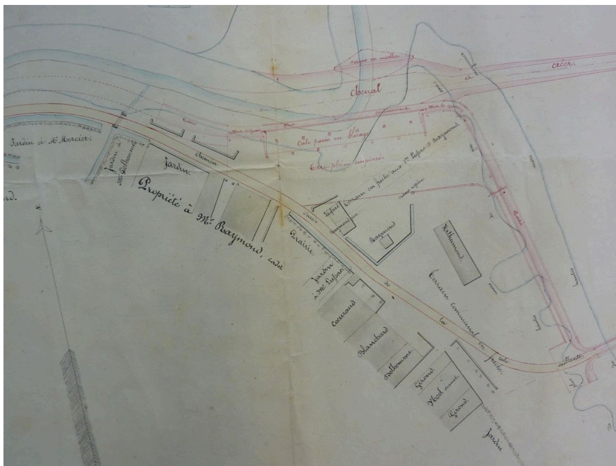
Plan du port indiquant les travaux à effectuer pour son amélioration, 25 janvier 1854 : détail.
