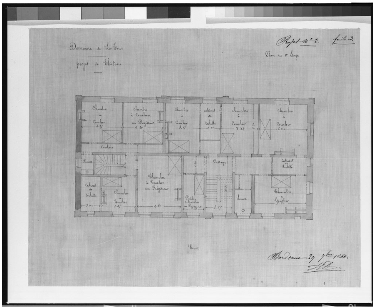
Projet de château, projet n°2 : plan du 1er étage, feuille 3, par Henri Duphot, 29 novembre 1860 (conservé au château?).
