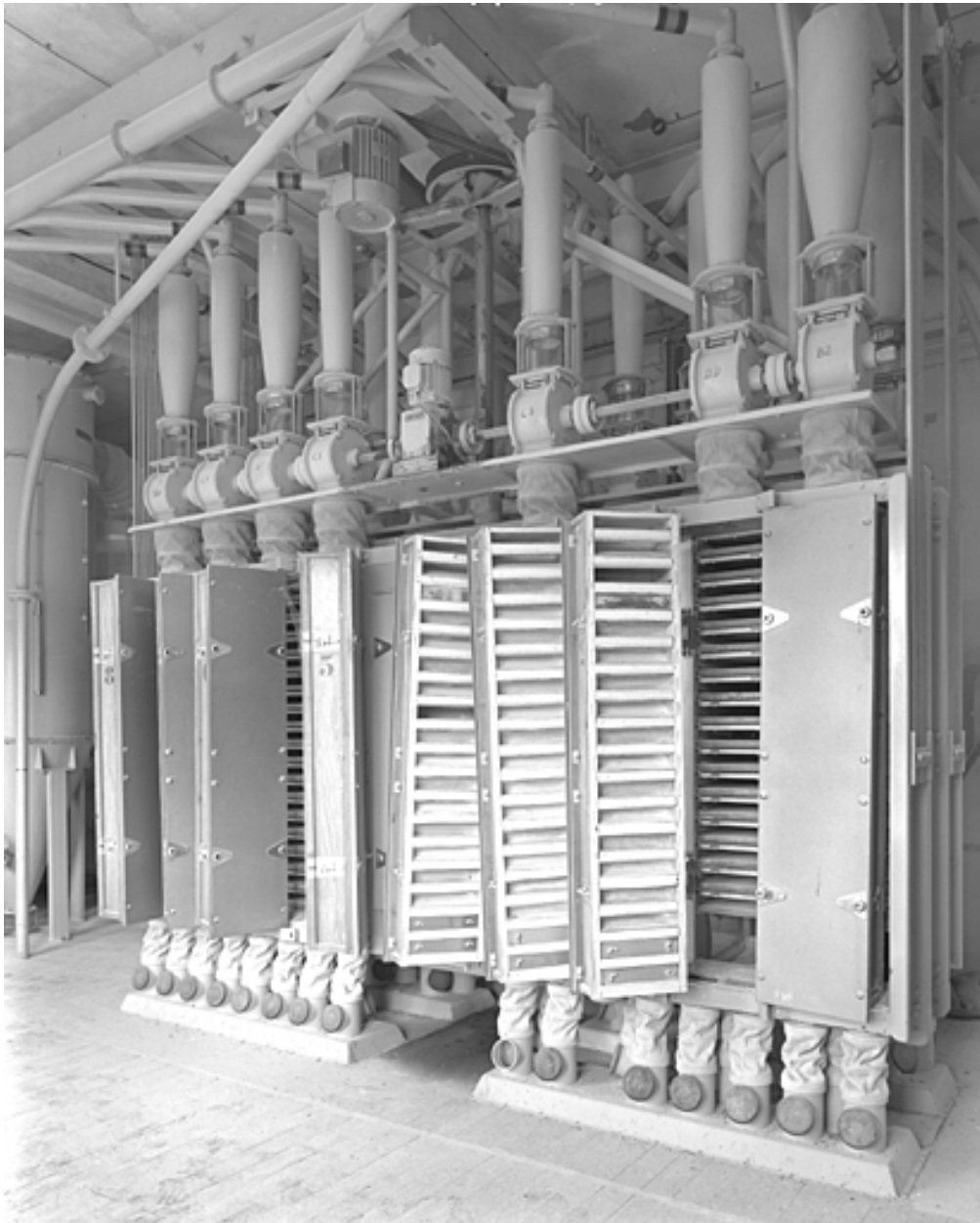
Troisième étage de la minoterie : plansichter pendulaire Buhler de 1965.
