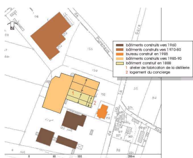
Plan masse, plan schématique des toitures. Dess. Zoé Lambert IVR54_19971709008NUDA
