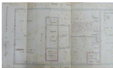
Projet de construction d'une mairie auprès de l'école ; plan en 1896. Phot. Pascale Moisson, Autr. Louis Girard IVR75_20211702085NUCA
