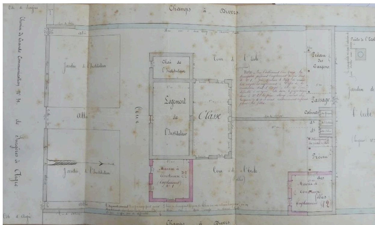
Projet de construction d'une mairie auprès de l'école ; plan en 1896.
