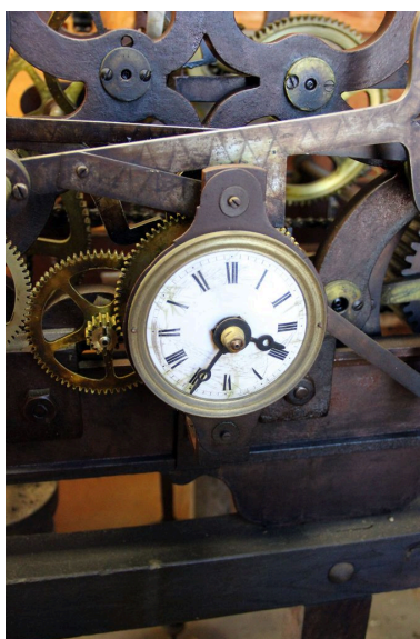
Détail du cadran émaillé.
