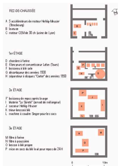
Plan schématique des différents niveaux, avec mention des machines.
