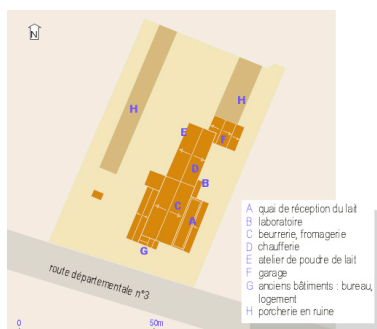
Plan masse, plan schématique des toitures. Dess. Zoé Lambert IVR54_20047900060NUDA
