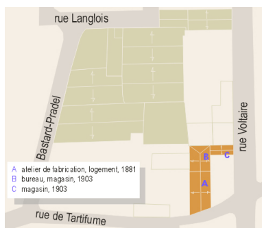
Plan masse, plan schématique des toitures. Dess. Zoé Lambert IVR54_20047900046NUDA
