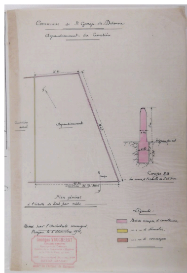
Plan extrait du devis établi en 1911 par Georges Vaucheret, architecte, pour l'agrandissement du mur de clôture. Phot. Yannis (reproduction) Suire IVR54_20141709390NUCA
