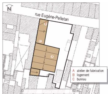
Plan masse, plan schématique des toitures. Dess. Zoé Lambert IVR54_20001707830NUDA
