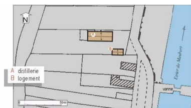
Plan masse, plan schématisé des toitures. Dess. Zoé Lambert IVR54_20011700287NUDA
